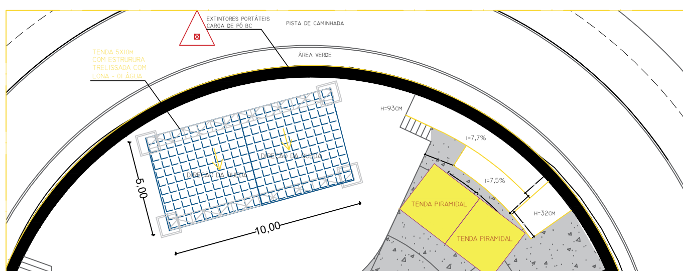
TENTA DO ANFITEATRO
