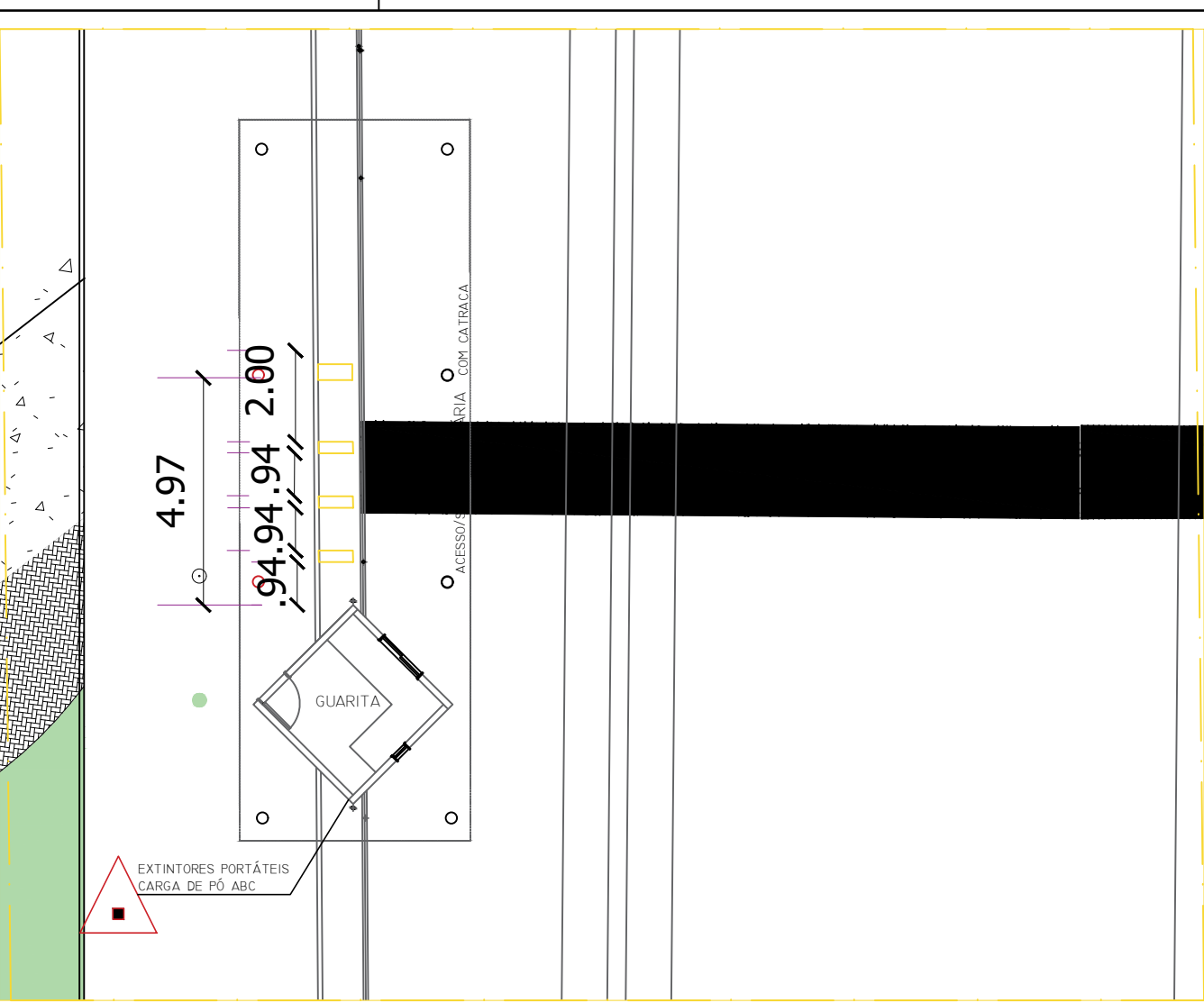
DETALHAMENTO DO ACESSO DO SHOPPING
