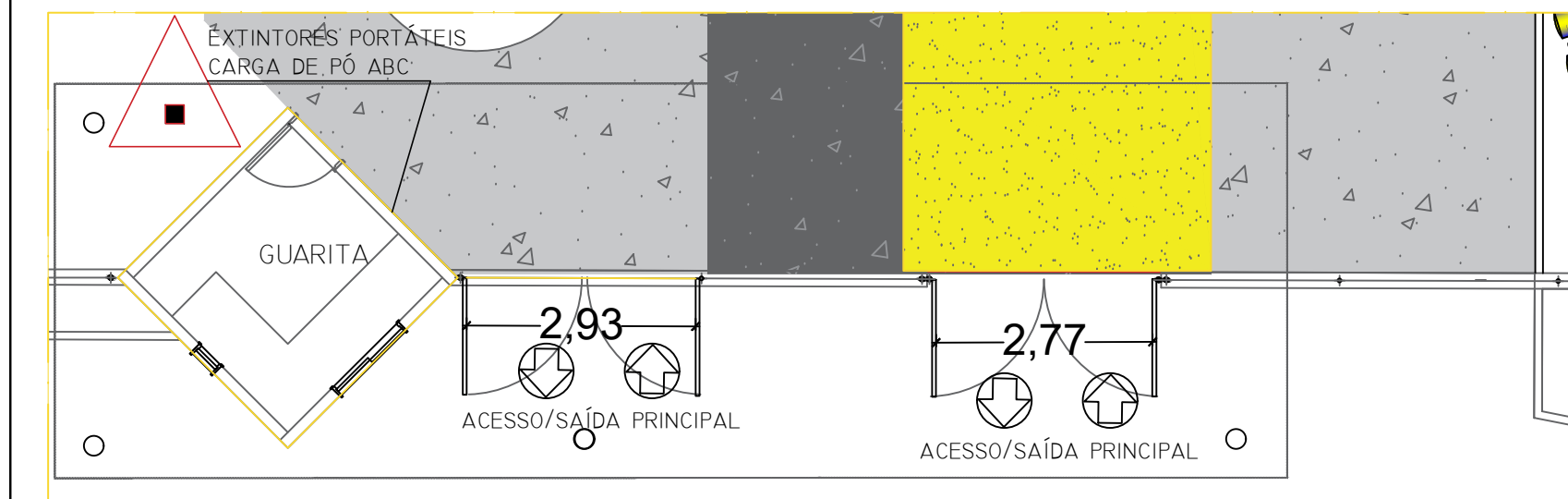
DETALHAMENTO DO ACESSO PRINCIPAL
