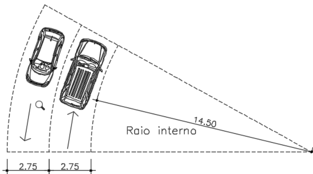
Figura 02 – Desenho exemplificando a curva com o raio interno de 14, 50 m.
