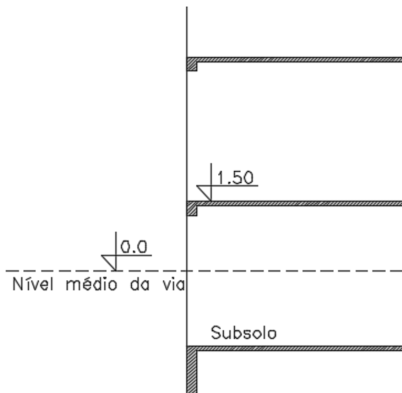
Figura 02 – Exemplo de nível do subsolo semienterrado.
