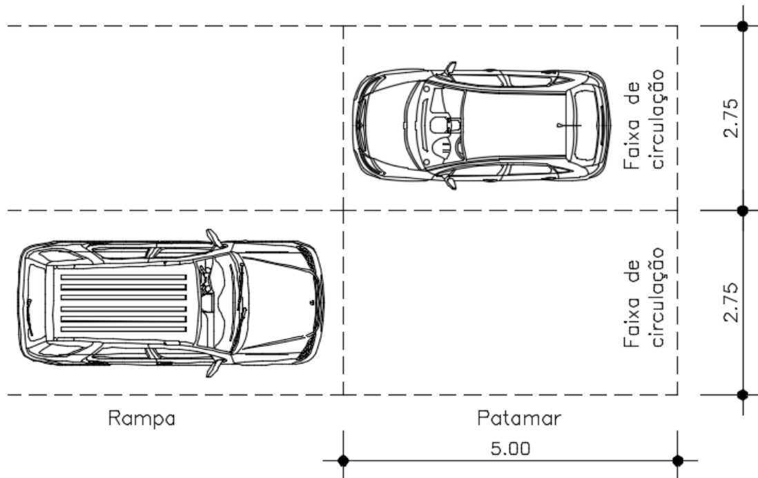
Figura 03 – Desenho utilizando as duas faixas de 2,75 m e o patamar mínimo de 5,0 m.
