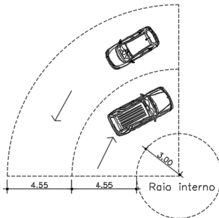
Figura 01 – Desenho exemplificando a curva com o raio interno de 3 m.
